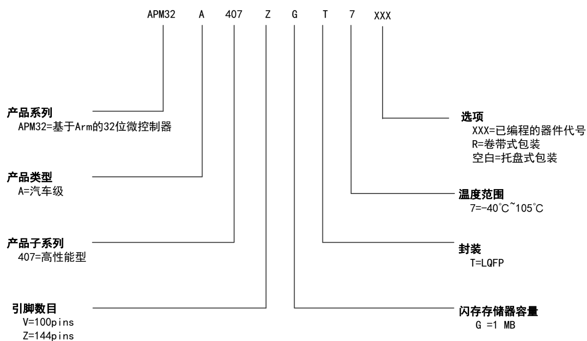
图 21 APM32A407xGT7 系列订货信息图
