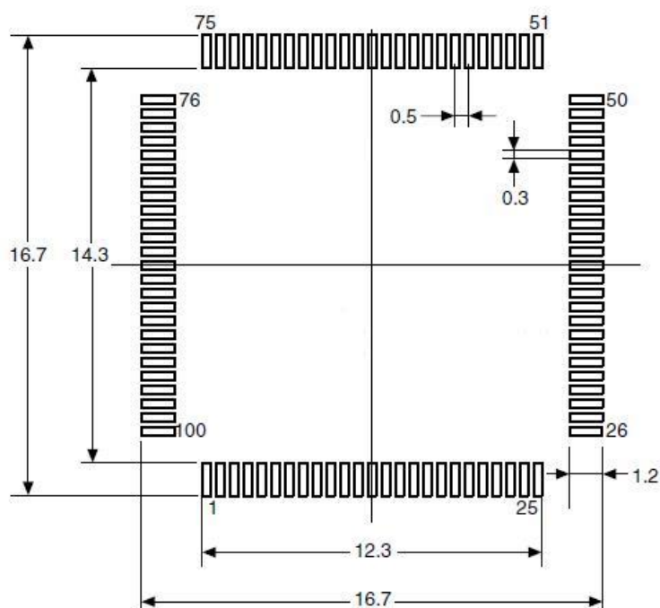
图 18 LQFP100 – 100 引脚，14 x 14mm 焊接 Layout 建议
