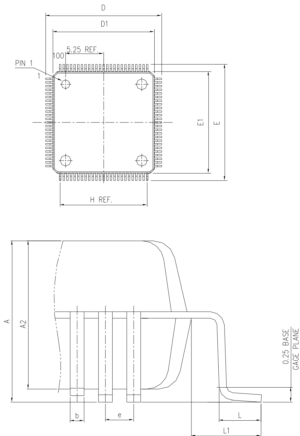
图 17 LQFP100 封装图
