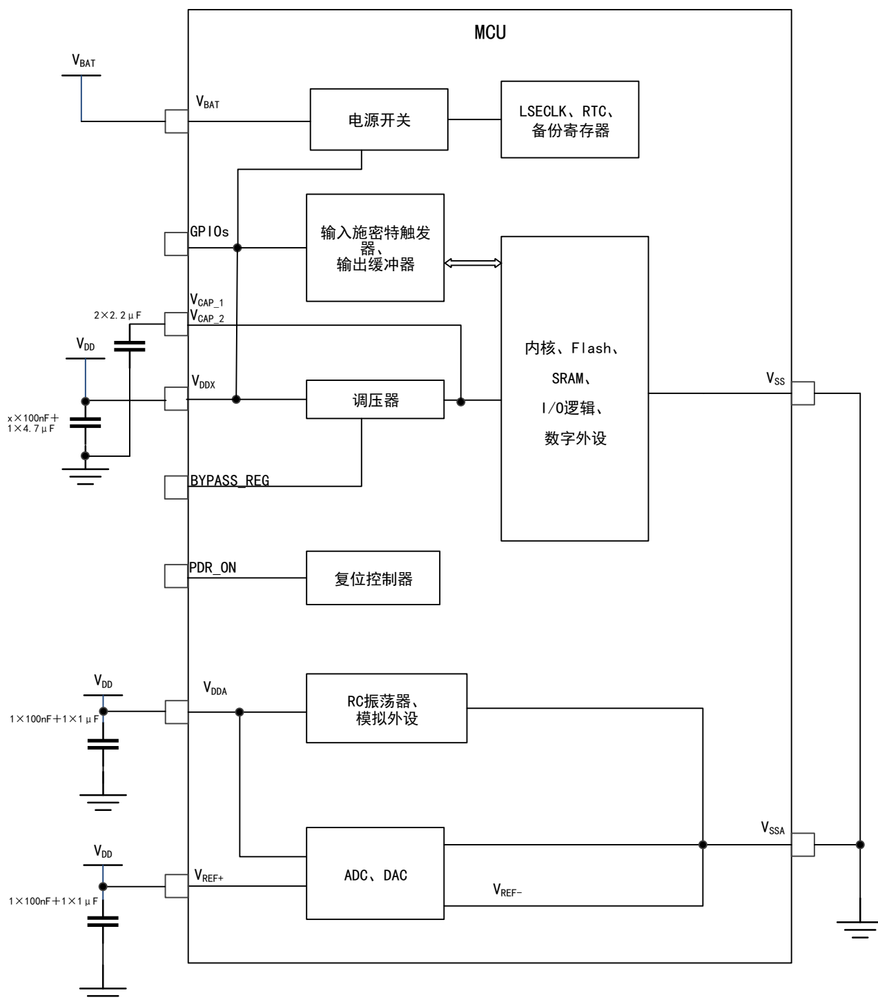
图 5 电源方案
